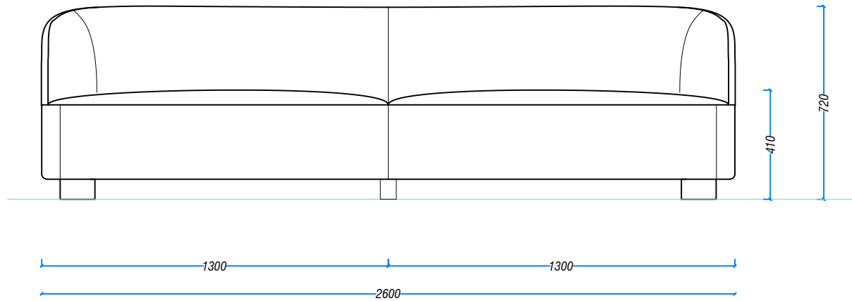
PROSPETTO FRONTALE
